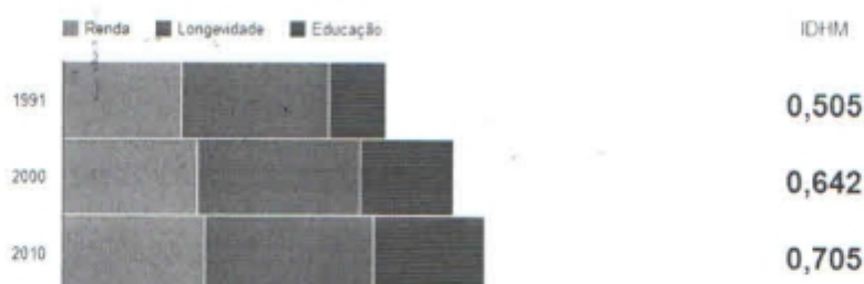
Gráfico 6 - IDHM
